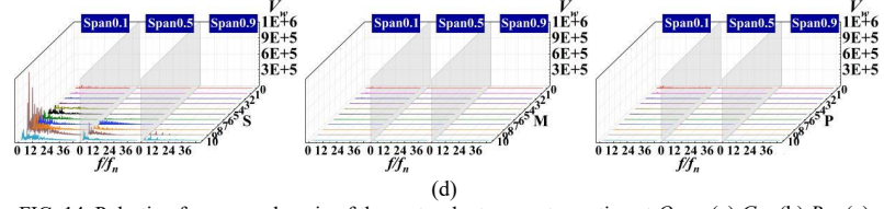
FIG. 14. Pulsation frequency domain of the enstrophy transport equation at Q_{BEP} : (a) G_\omega ; (b) R_\omega ; (c) C_\omega ; (d) V_\omega .
